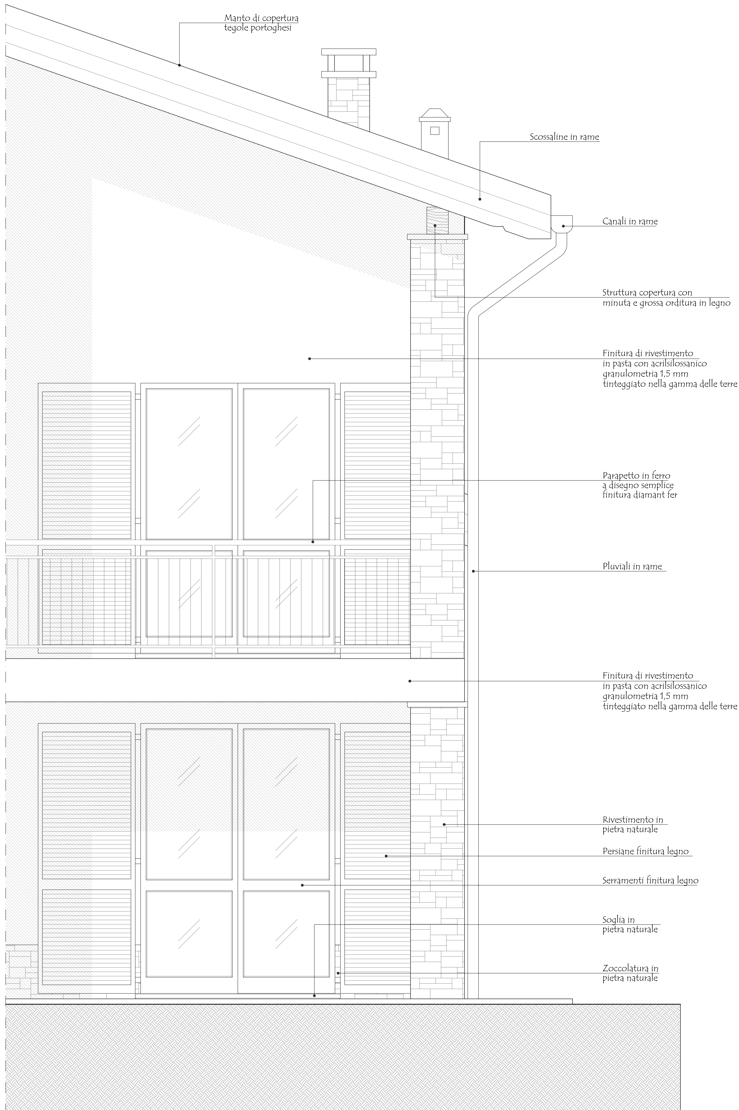
PARTICOLARE PROSPETTO
