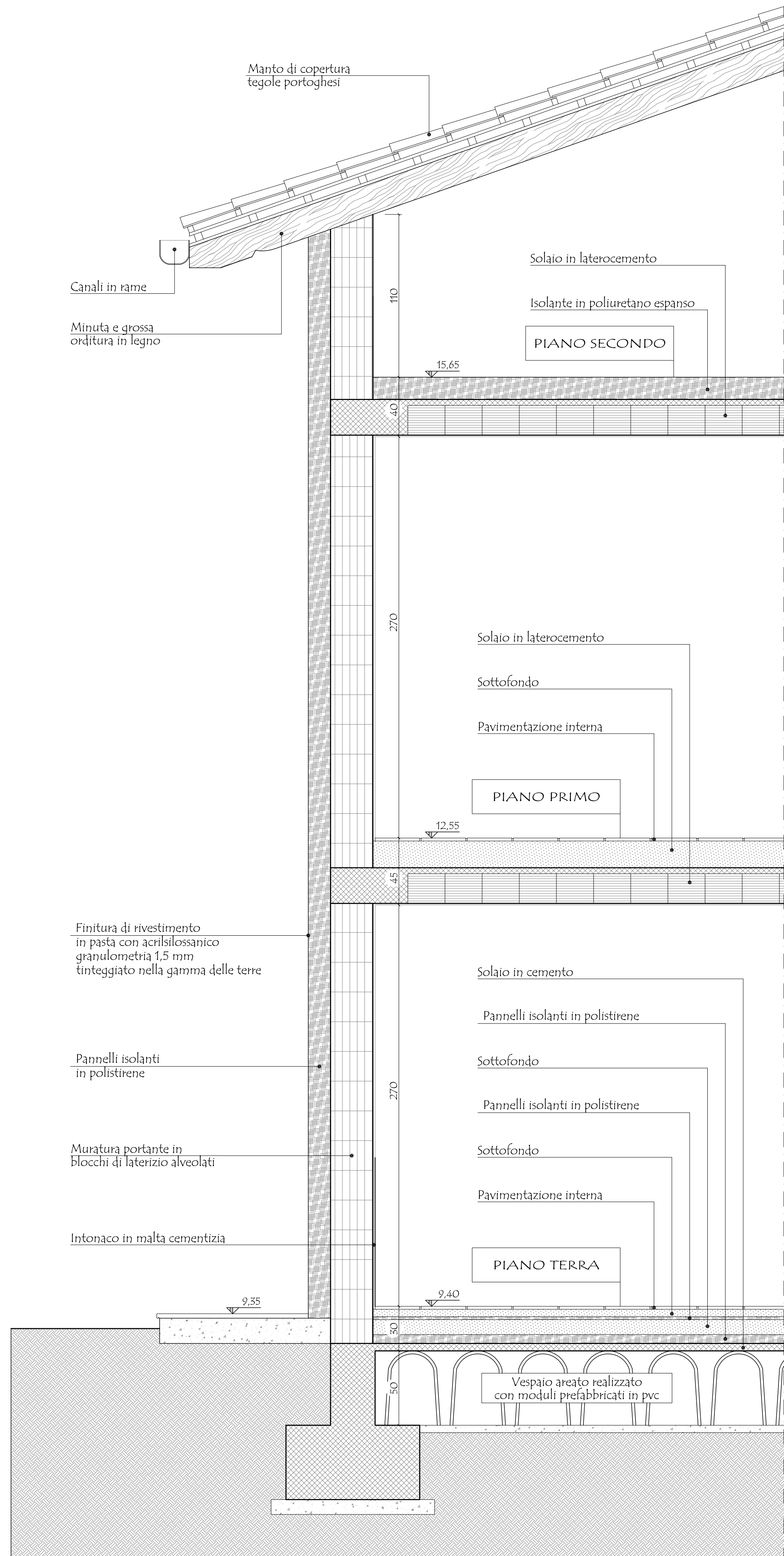
PARTICOLARE SEZIONE
