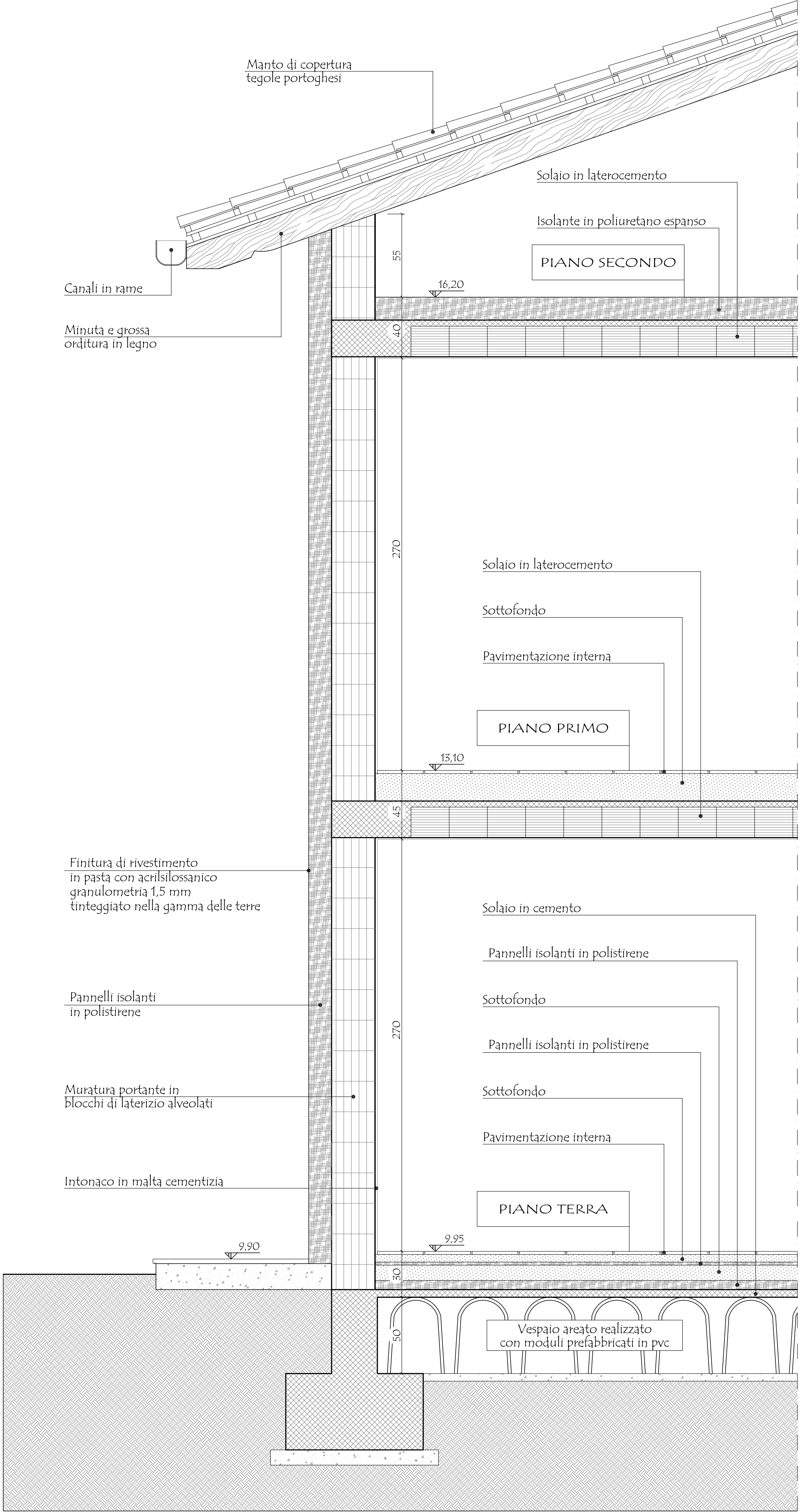
PARTICOLARE SEZIONE
