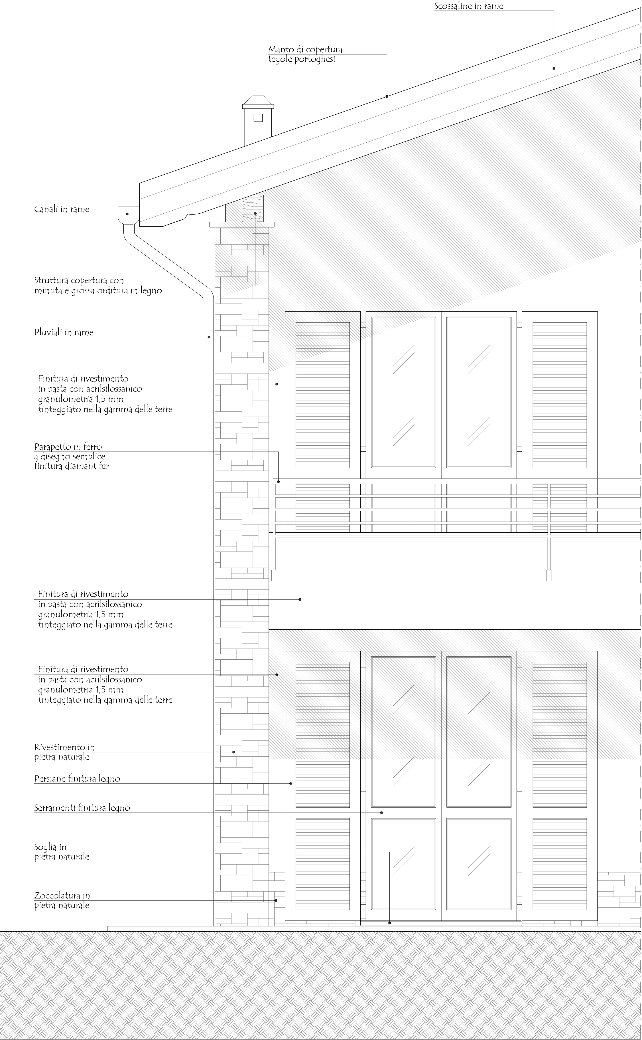
PARTICOLARE PROSPETTO
