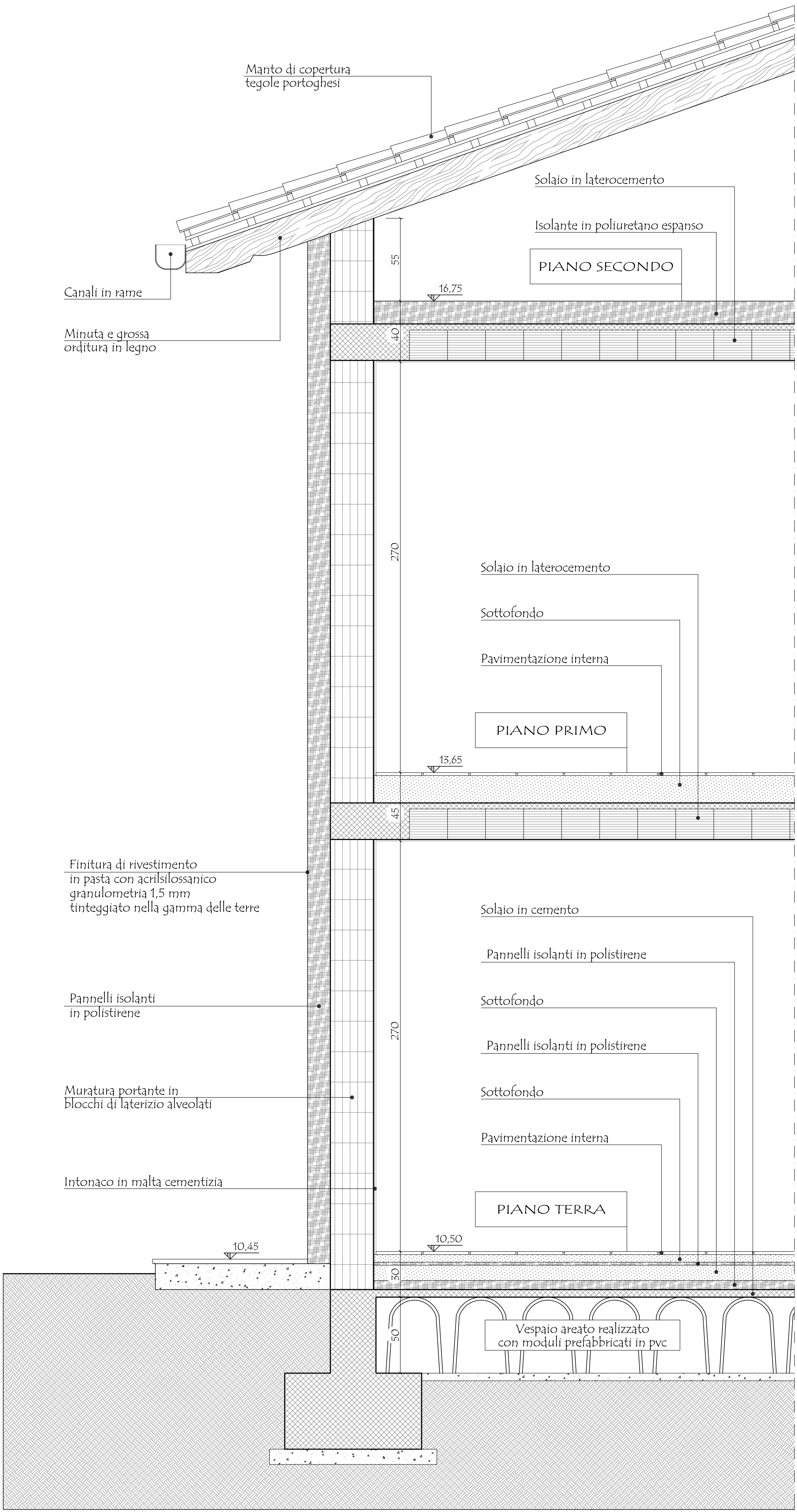
PARTICOLARE SEZIONE
