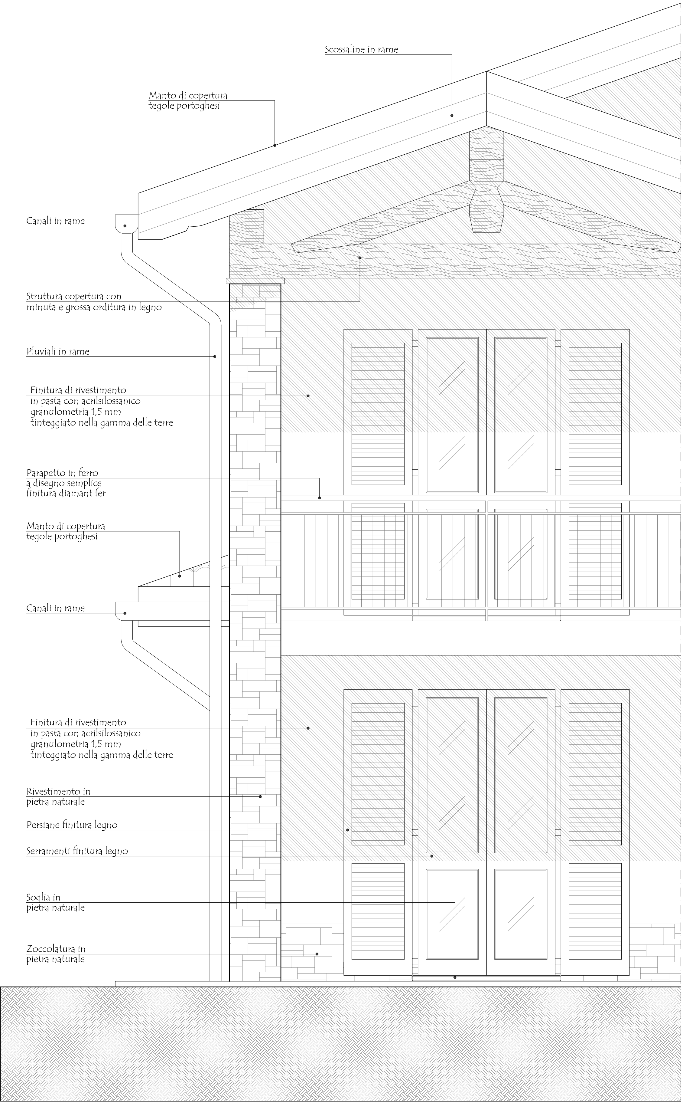
PARTICOLARE PROSPETTO
