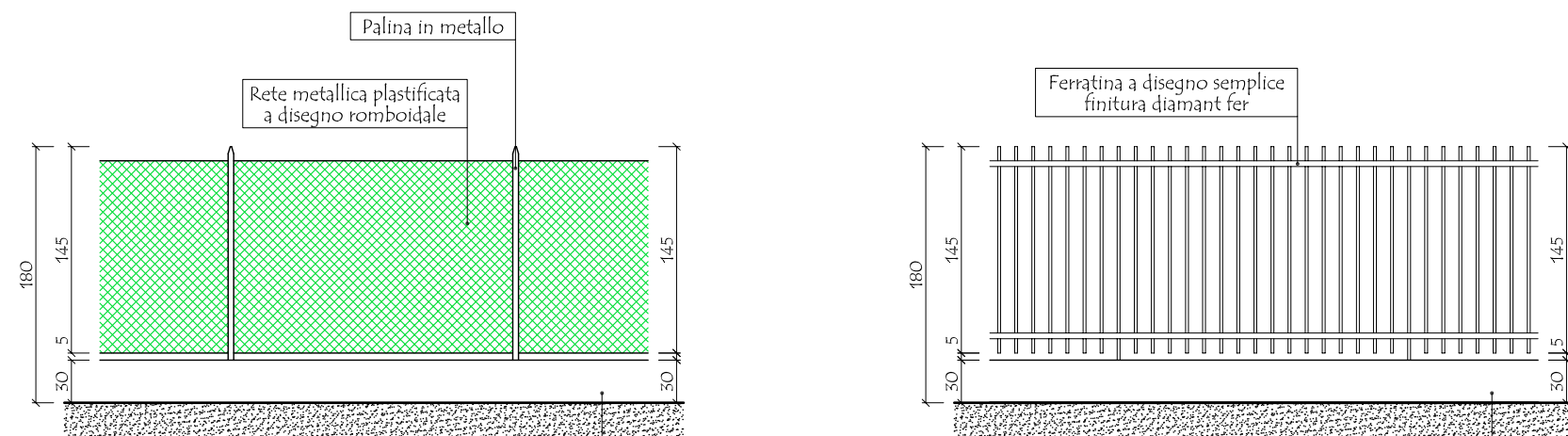
PARTICOLARE RECINZIONE MURETTO SORMONTATO DA PALI E RETE A-B B-C C-D D-E F-G G-H J-K L-M M-N D-O O-P Q-R V-W SCALA 1:50
