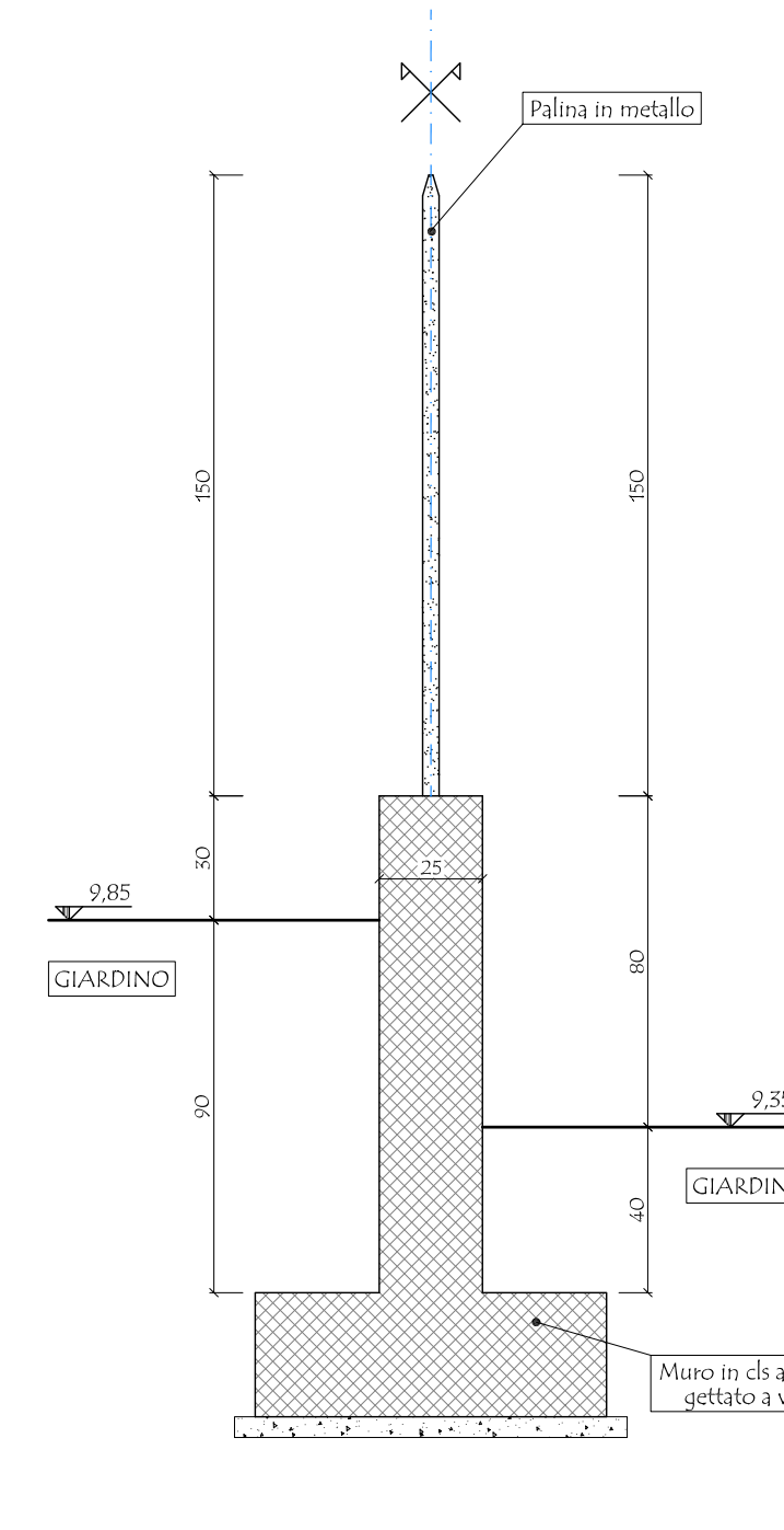
TRATTO DI RECINZIONE Q-R SEZIONE 6-6' - SCALA 1:20
