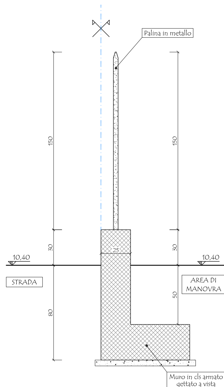
TRATTO DI RECINZIONE A-B B-C SEZIONE 1-1' - SCALA 1:20
