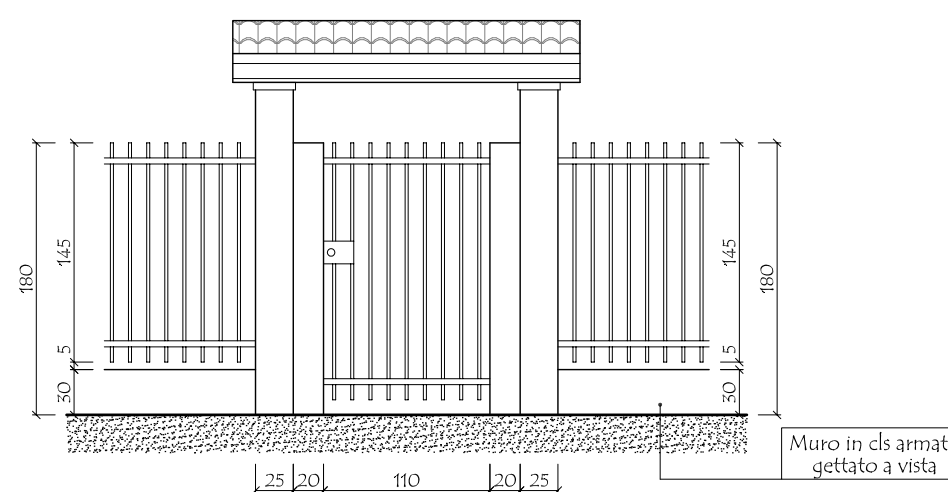
PARTICOLARE CANCELLO PEDONALE SCALA 1:50
