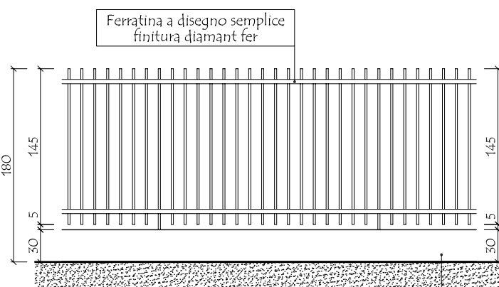
PARTICOLARE RECINZIONE MURETTO SORMONTATO DA FERRATINA X-Y Y-Z R-S S-T T-U H-I I-J SCALA 1:50
