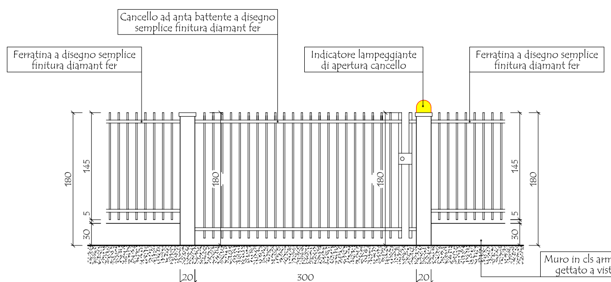
PARTICOLARE CANCELLO CARRAIO SCALA 1:50
