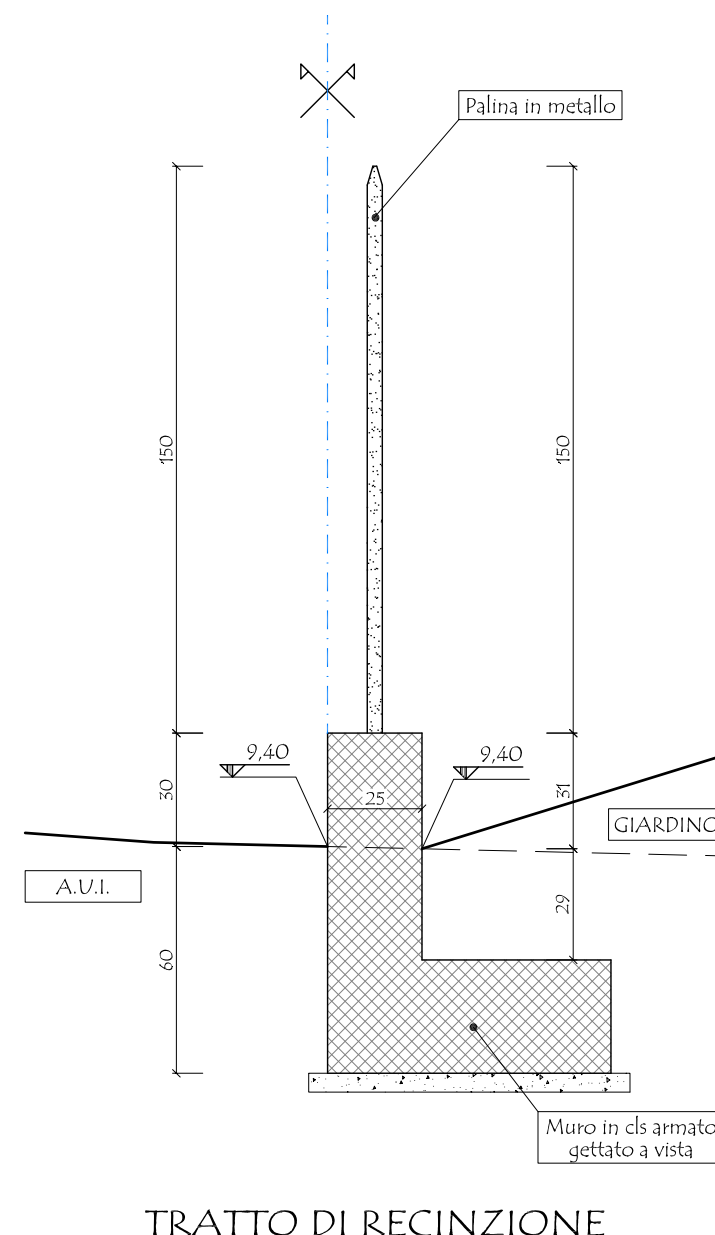
TRATTO DI RECINZIONE C-D D-O O-P V-W SEZIONE 2-2' - SCALA 1:20
