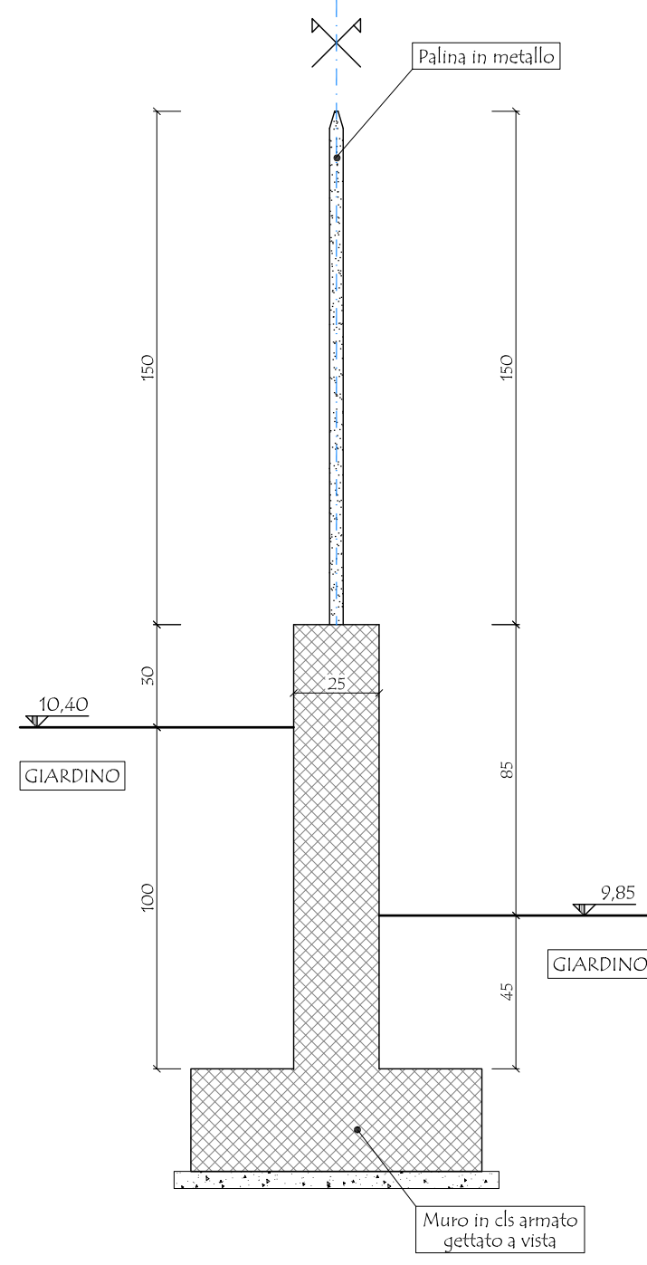
TRATTO DI RECINZIONE D-E SEZIONE 5-5' - SCALA 1:20
