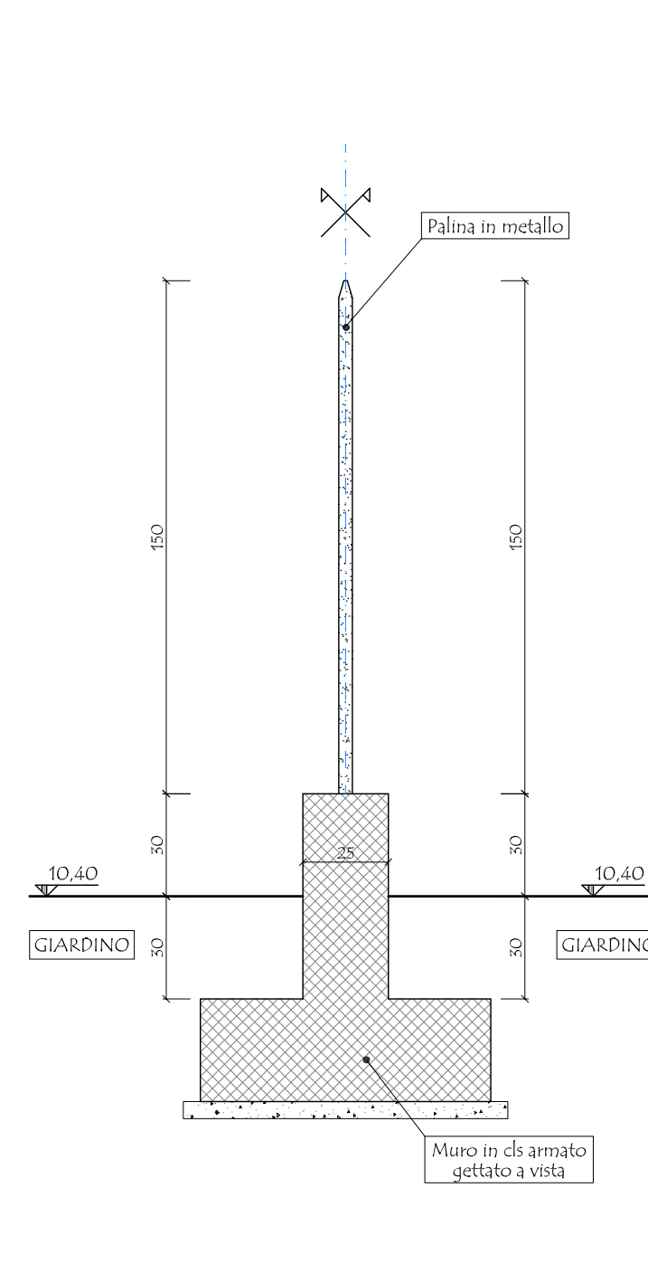
TRATTO DI RECINZIONE F-G G-H J-K L-M M-N SEZIONE 7-7' - SCALA 1:20
