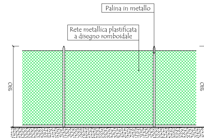
PARTICOLARE RECINZIONE PALI E RETE P-Q W-X SCALA 1:50
