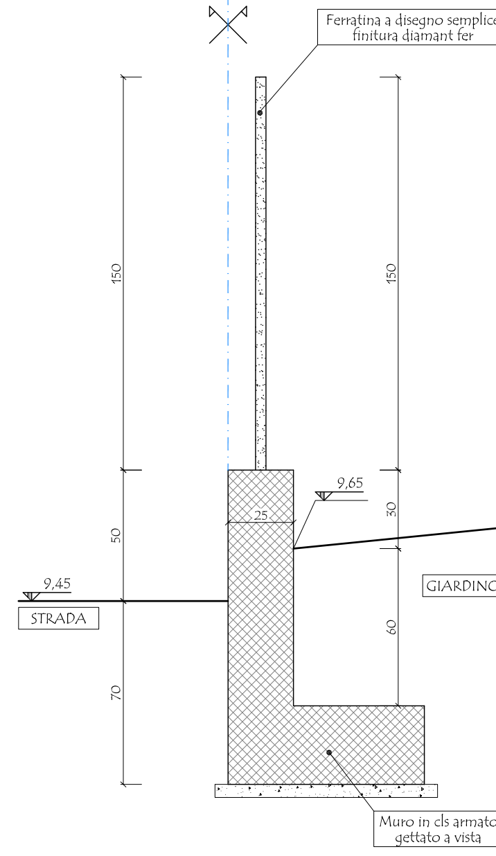
TRATTO DI RECINZIONE X-Y Y-Z R-S S-T T-U H-I I-J SEZIONE 4-4' - SCALA 1:20
